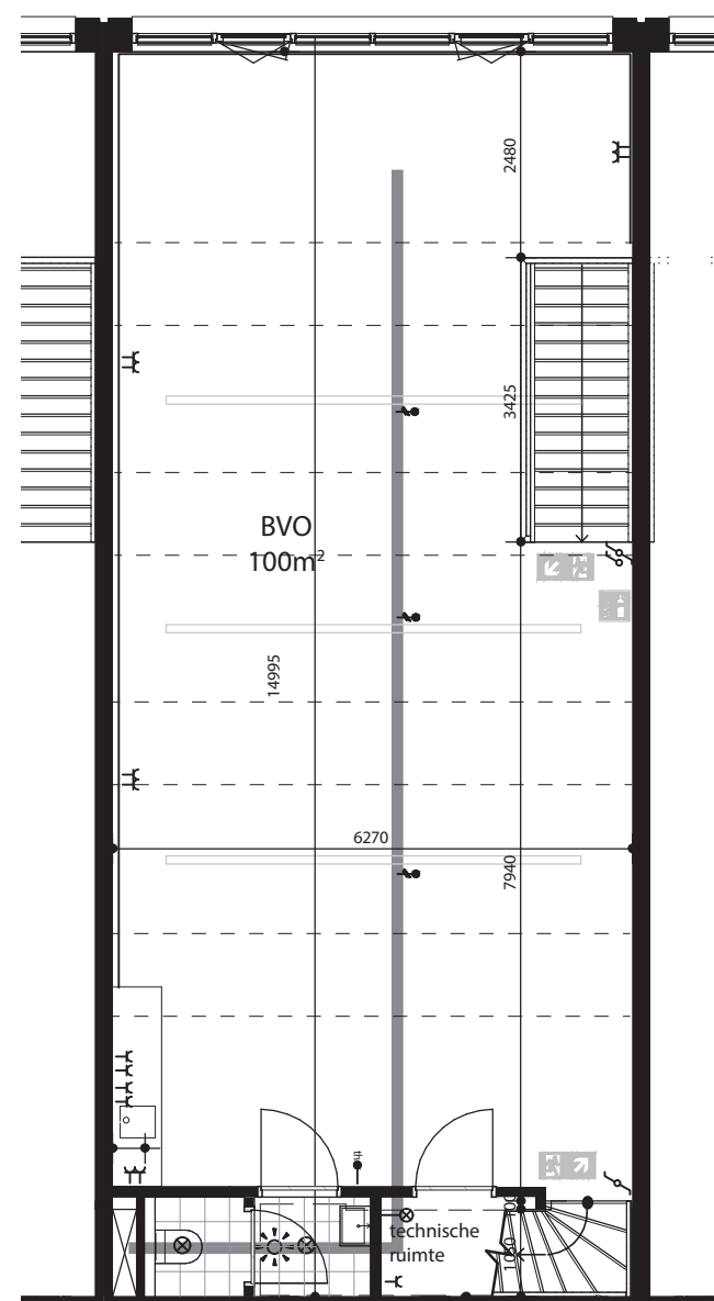
2 Eerste verdieping 1:100
