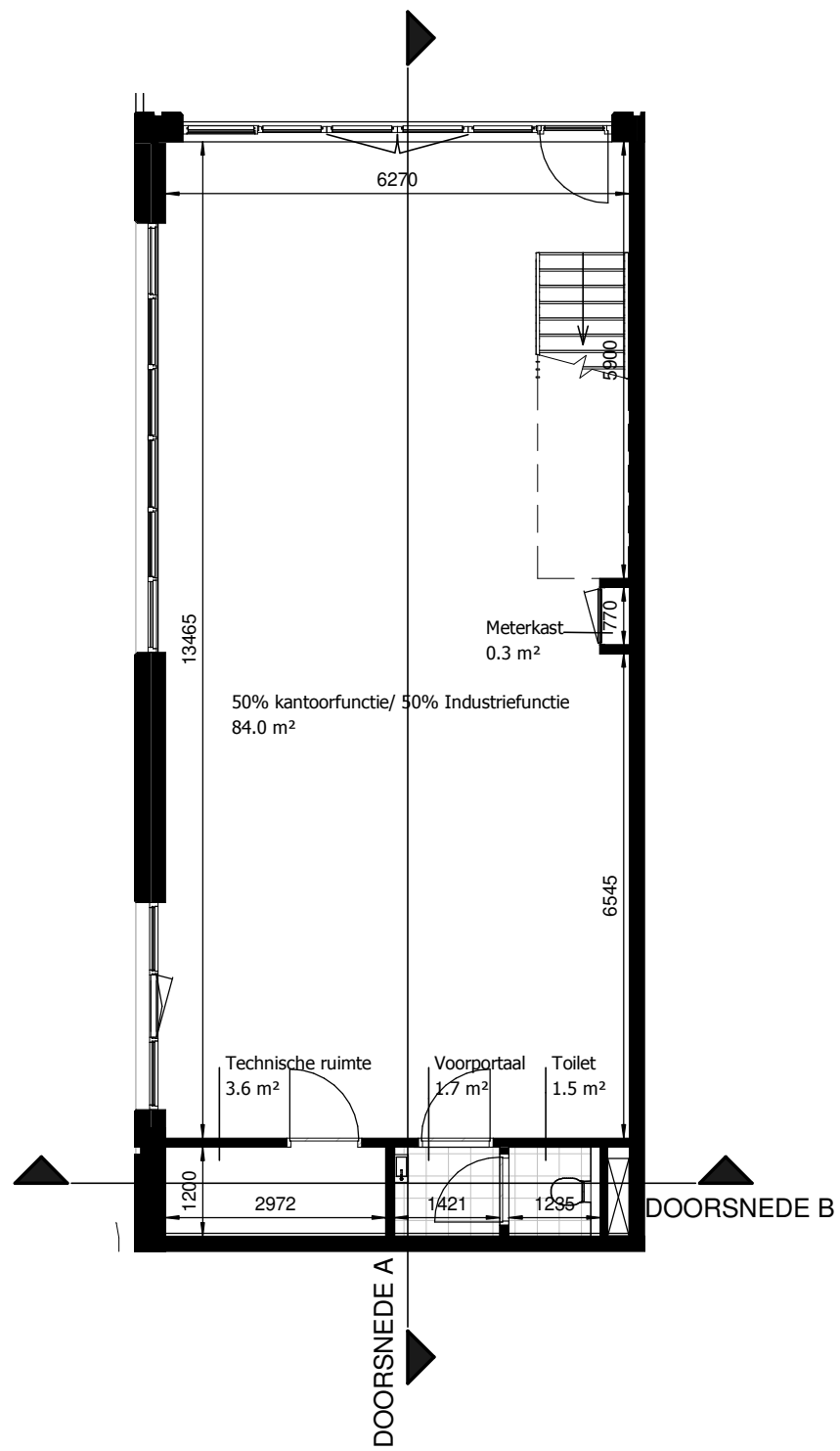
Begane Grond 1:100
