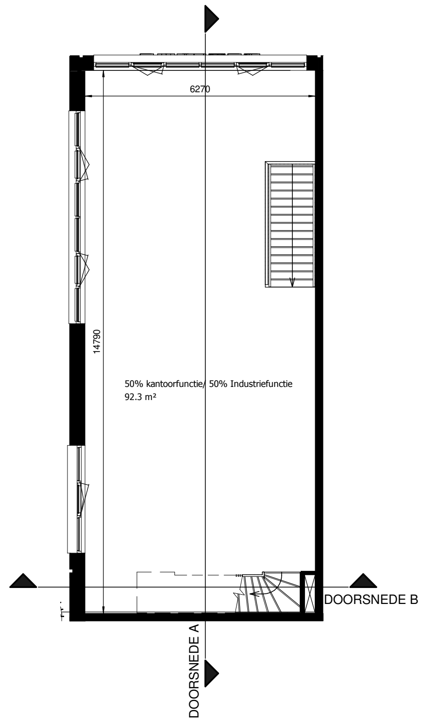
1e Verdieping 1:100
