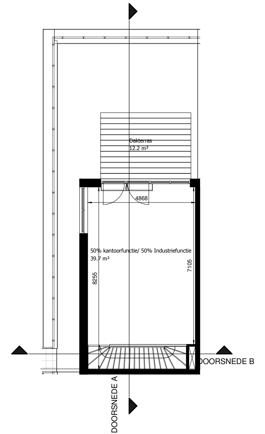
2e Verdieping 1:100
