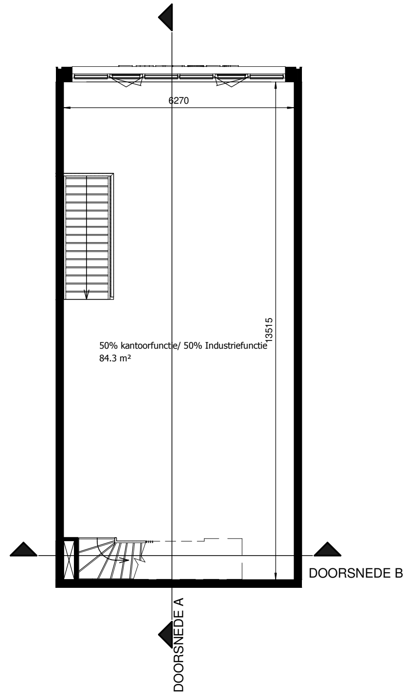
1e Verdieping
