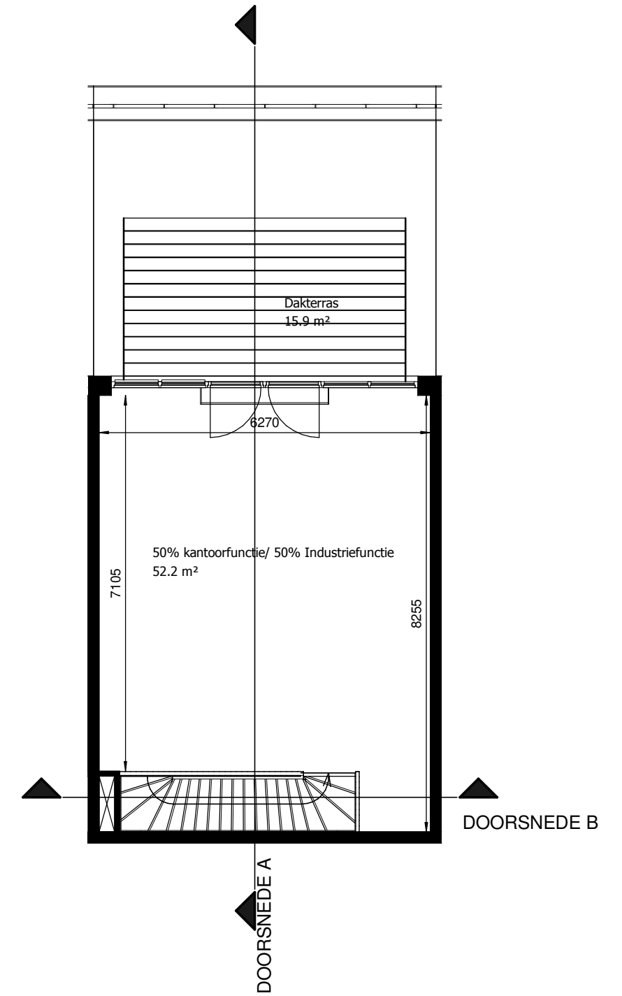
2e Verdieping
