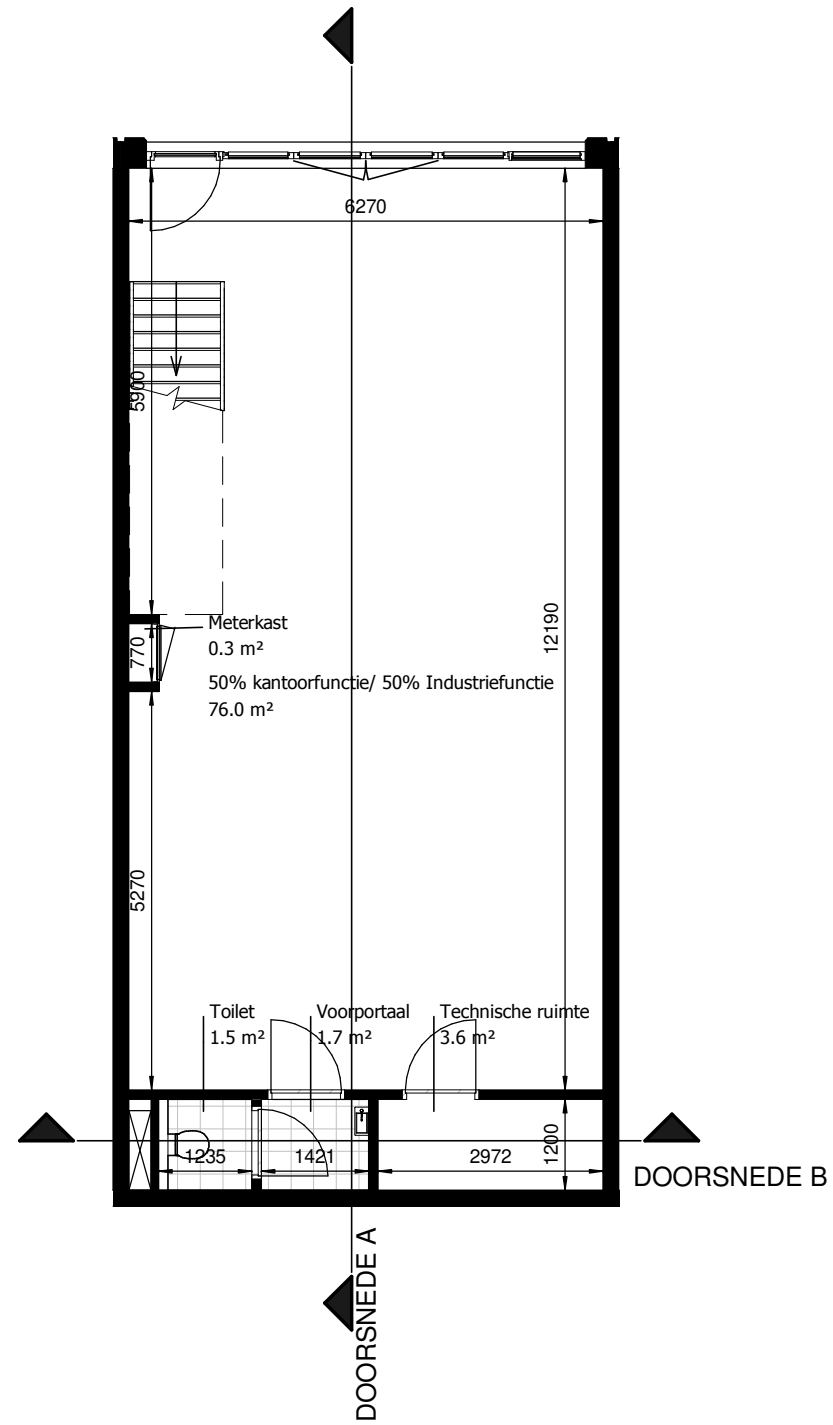
Begane Grond
